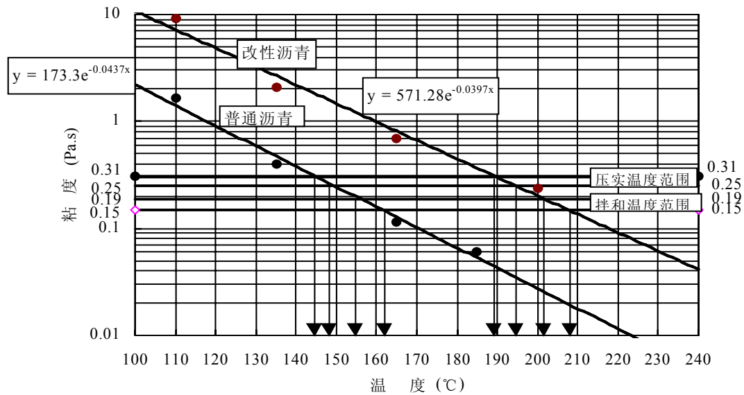
图 5.2.4 普通沥青及改性沥青的粘温曲线
