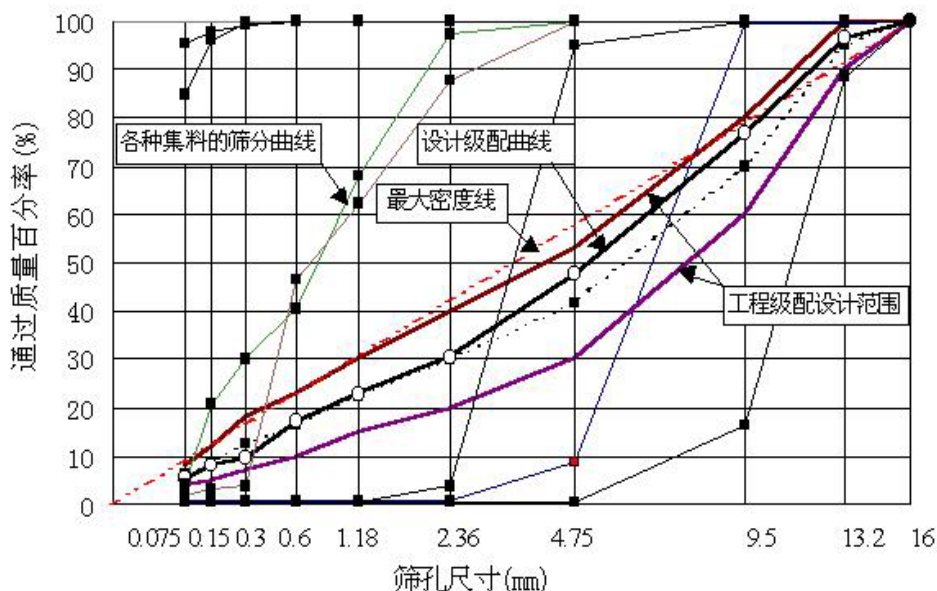
图 B.4.2 矿料级配曲线示例
