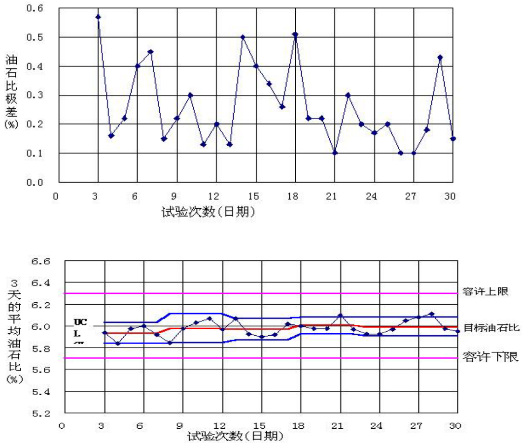
图 F.0.3 动态质量管理图 ( \bar{X}-R 管理图) 示例(油石比, %)
