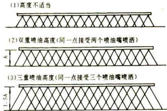
图 6.2.6 沥青洒布车喷油嘴的高度
