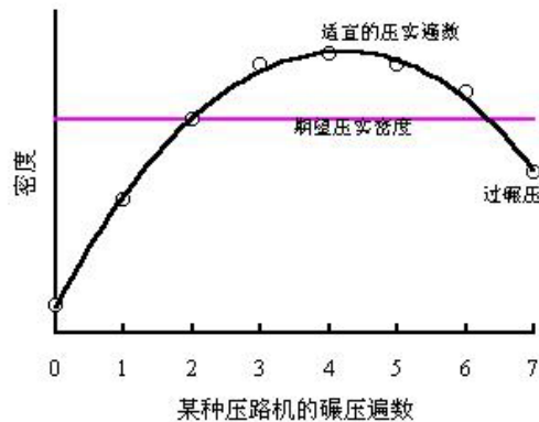
图 11.4.8-2 沥青路面的过碾压
