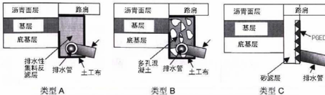
图 10.7.1 AASHTO 沥青路面结构层边缘排水方案
