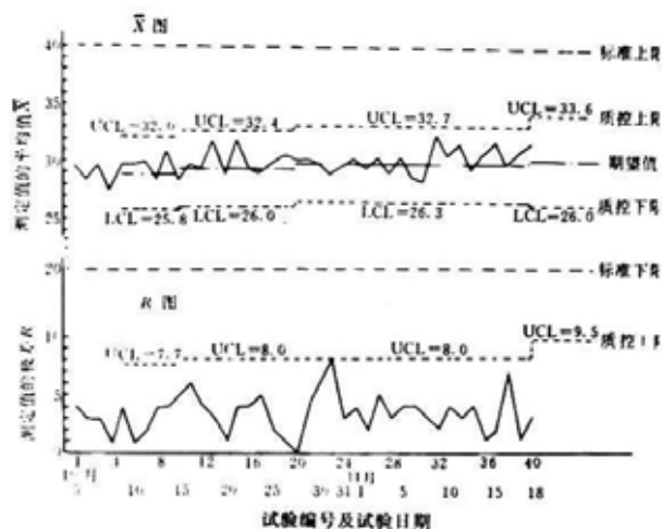
图 F.0.3-1 工程质量指标管理图示例(流值, mm)
